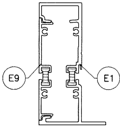
JAMB 'J1'
